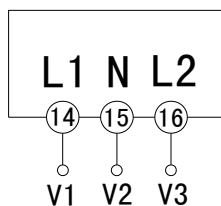
图 8：控制板电源接线图
