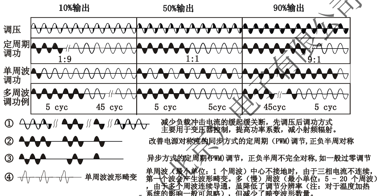
图 10 调压调功的负载电压电流波形对比
